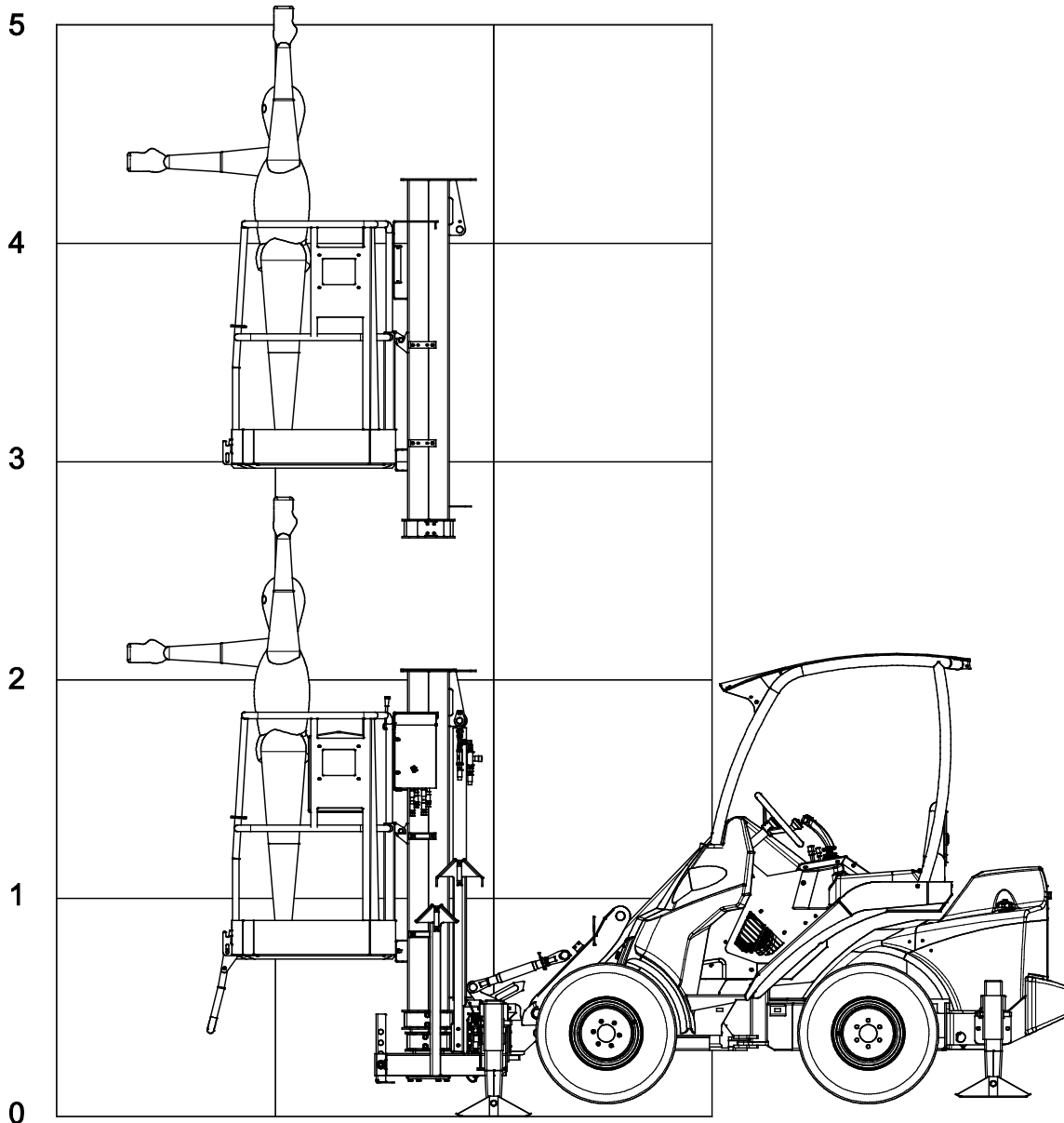
Figura 4. Gráfico de alcance de la plataforma de acceso Leguan 50
