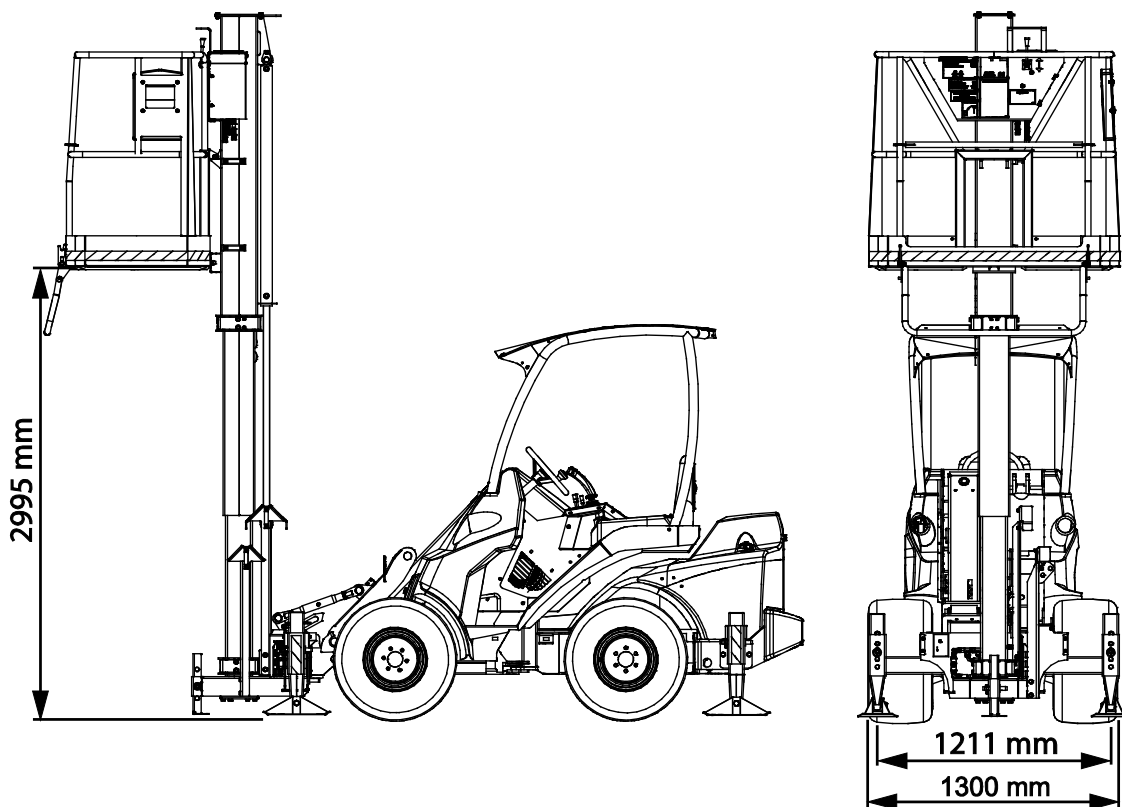
Figura 2. Plataforma de acceso LEGUAN 50 montada en la minicargadora Avant
